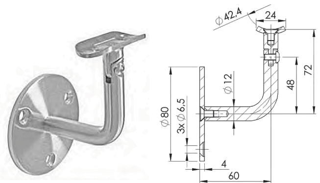
MV-016 SIENINIS TURĖKLŲ TVIRTINIMAS (reguliuojamas)
