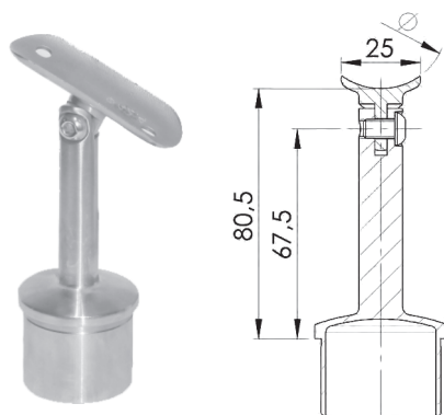
MV-034.2 ŽVAKĖ (reguliuojama)
