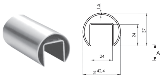
MV-040 U PROFILIS
