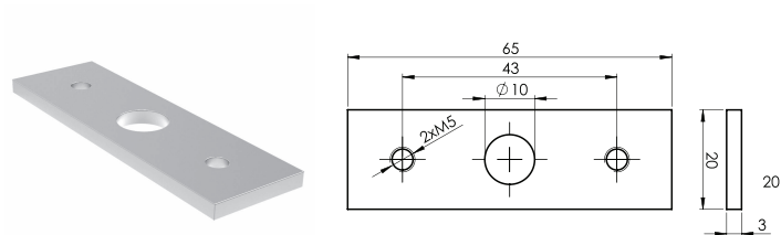
MV-060.2 LAIKIKLIS LED TURĖKLUI
