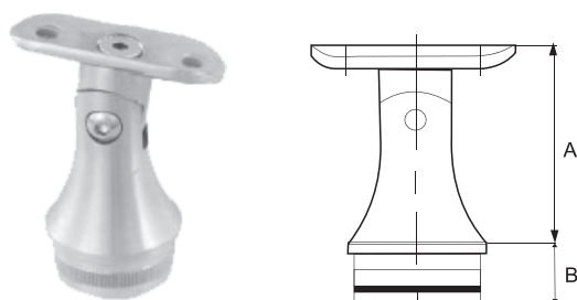
MV-030 ŽVAKĖ (reguliuojama)
