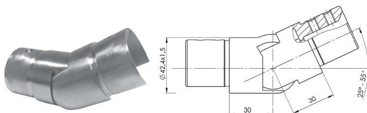
MV-041 U PROFILIS ALKŪNĖ (reguliuojama)
