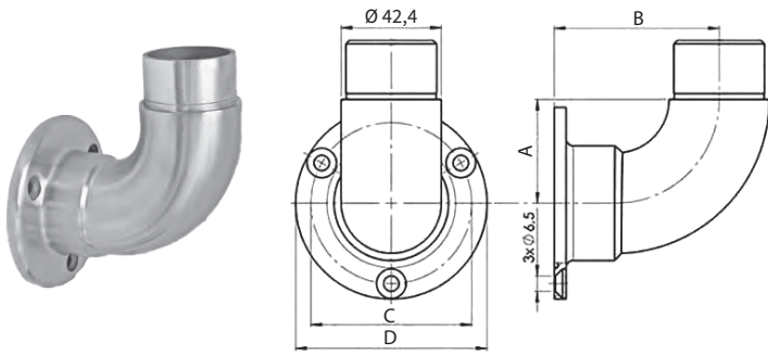
MV-013.1 SIENINIS VAMZDŽIO TVIRTINIMAS
