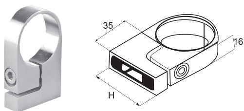
MV-037 SIENINIS VAMZDŽIO TVIRTINIMAS (ŽIEDAS)
