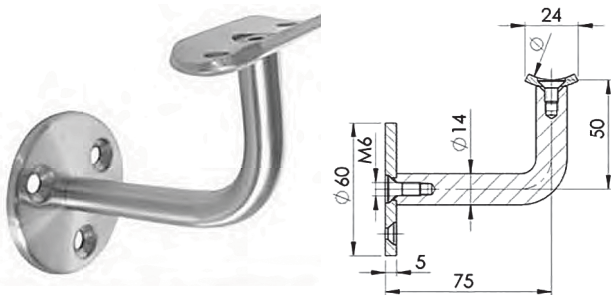
MV-015 SIENINIS TURĖKLŲ TVIRTINIMAS
